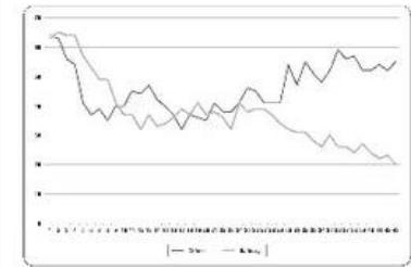
Figure 3. Comparaison de la cote de confiance de Chirac au cours de son premier mandat et de Sarkozy au cours de son mandat.
